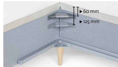
▶ Angolare regolabile in 2 altezze Adjustable corner brackets in 2 heights
